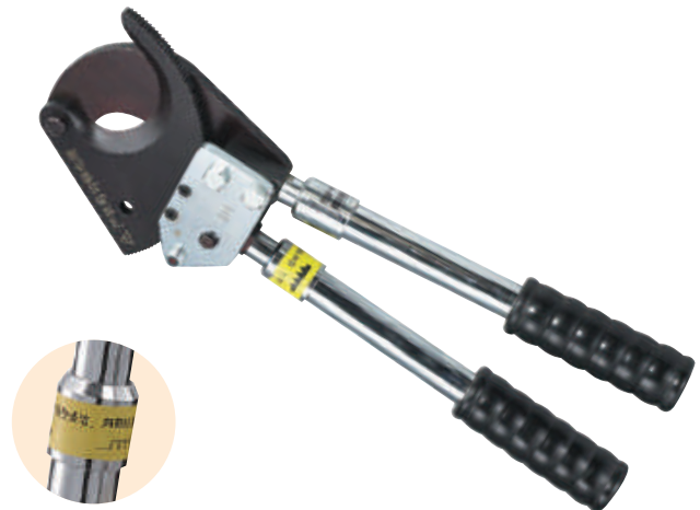
可伸缩手柄
